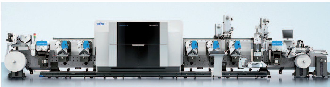
Die Gallus Labelfire bei Insignis verfügt über erweiterte Inline-Veredelungsprozesse, wie zum Beispiel Kaltfolien- und Siebdruck.
