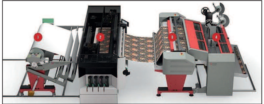
Die UVgel Wallpaper Factory ist eine vollautomatische Produktionslinie für digital bedruckte Tapeten und besteht aus Abrolleinheit, Drucker, Konfektionier und Ausgabeinheit.
