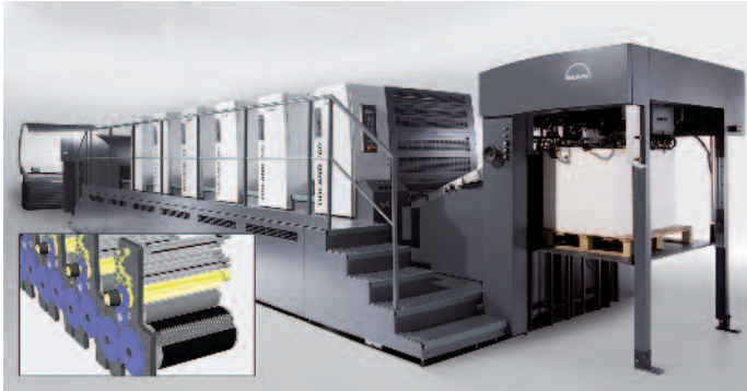
QuickChange-Module an der ROLAND 700 DirectDrive und an der ROLAND 700 HiPrint sorgen für drastische Einsparungen beim Rüstvorgang und der benötigten Makulatur.
