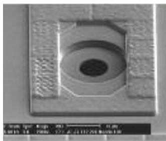
Vergrösserte Ansicht von Heizelement und Düsenöffnung.
