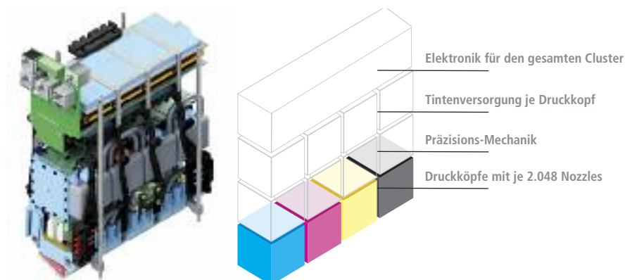
Die Basiskomponente aller Mouvent-Geräte – der Mouvent Cluster (ganz links und in der Schemazeichnung). Jeder einzelne autonome Cluster ist voll funktionsfähig. Die einzelnen Cluster können zu einer modularen, skalierbaren Matrix kombiniert
