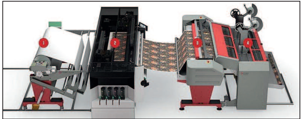
Die UVgel Wallpaper Factory ist eine vollautomatische Produktionslinie für digital bedruckte Tapeten und besteht aus Abrollereinheit, Drucker, Konfektionier und Ausgabeeinheit.
