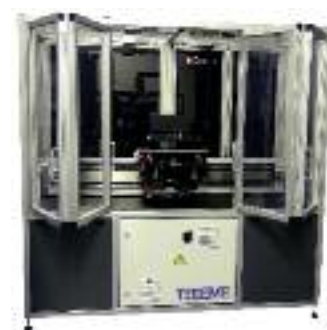
Das innovative Digitaldrucksystem Thiem LAB Digital ist für Single- und Multipassanwendungen geeignet und zeichnet sich durch eine hochpräzise Lineartechnologie sowie eine variable Druckkopfanzahl aus. Die Substratdicke (max. 50 mm) ist programmierbar.
